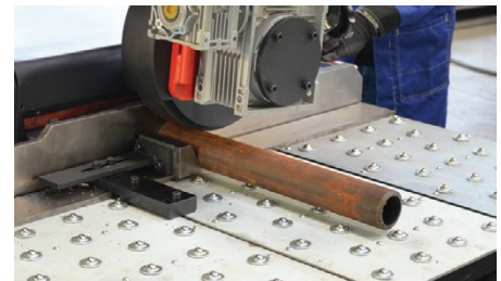
Possibility of pipe OD beveling
